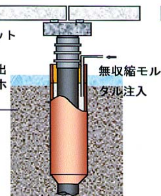
⑦無収縮モルタルの注入
