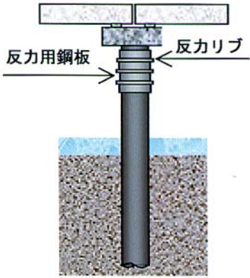
①反力用鋼板の設置
