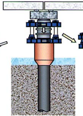
③補強鋼板の圧入
